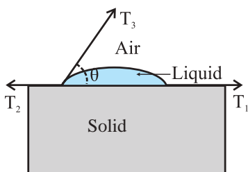
Fig. 2.20 (a): Acute angle.
