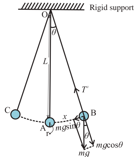
Fig.5.10: Simple pendulum.
